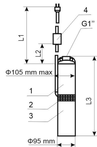
Obr.1 Rozměry a přípojovací rozměry 1 – čerpací díl, 2 – filter, 3 – elektrický motor, 4 – kondenzátorový box.
